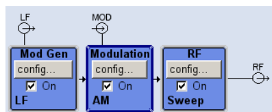
Fig. 4-2 : schéma fonctionnel du R&S SMB
